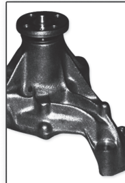
Correcta altura de ensamble a la maza 6.933" E.O. = 6.937" + 0.015"
