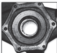
Maquinado descentrado del alojamiento de sello
